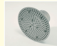
Siebreflektor Brause, Ø 150 mm Artikel-Nr.: 107.335
