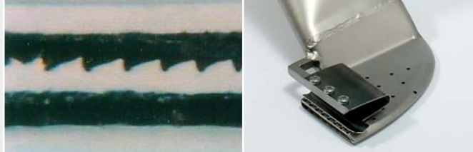
L'ugello „Grip“ brevettato permette di evitare il prelavaggio dei teli in TPO. (Accessorio)
